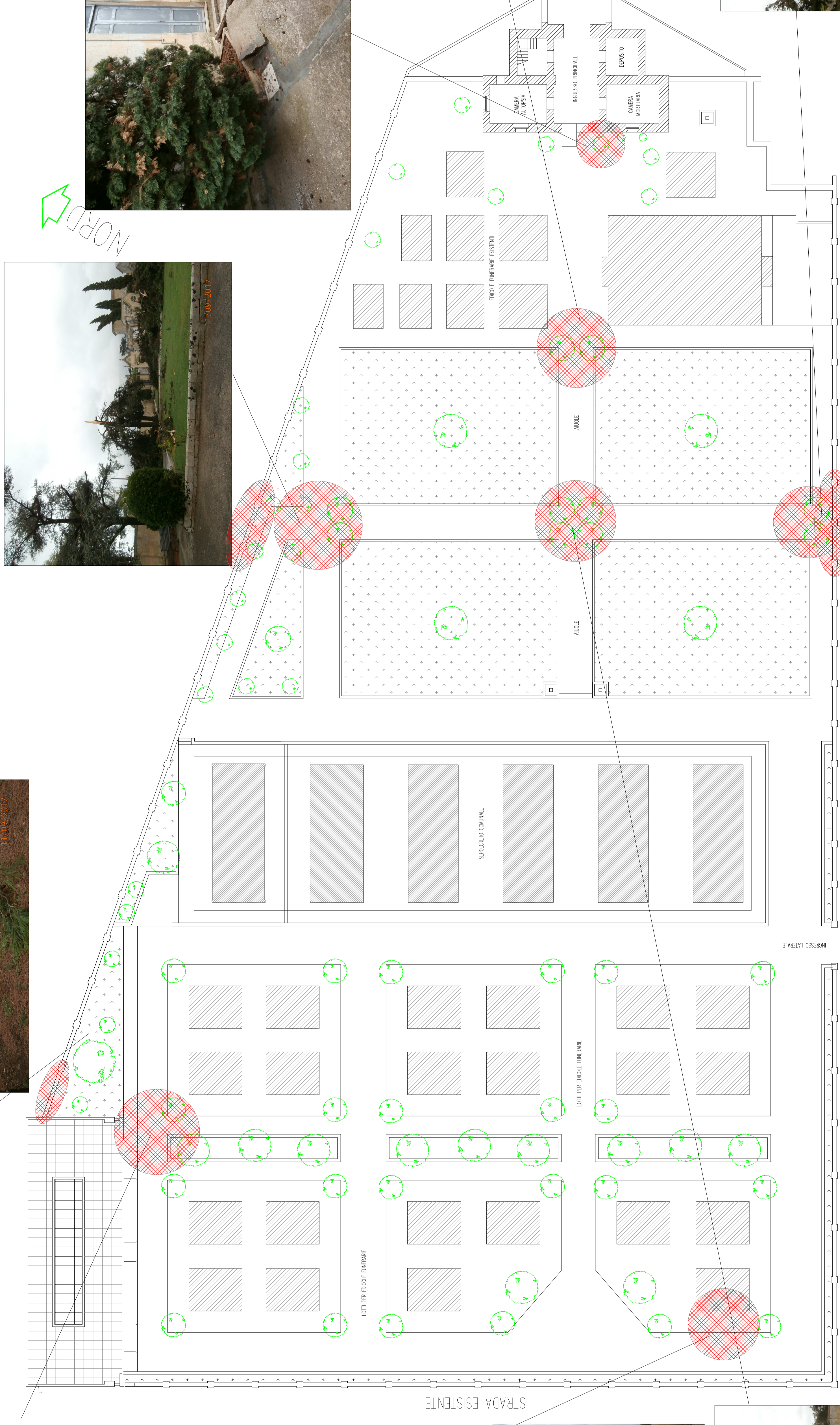
PLANIMETRIA GENERALE SCALA 1 : 200
