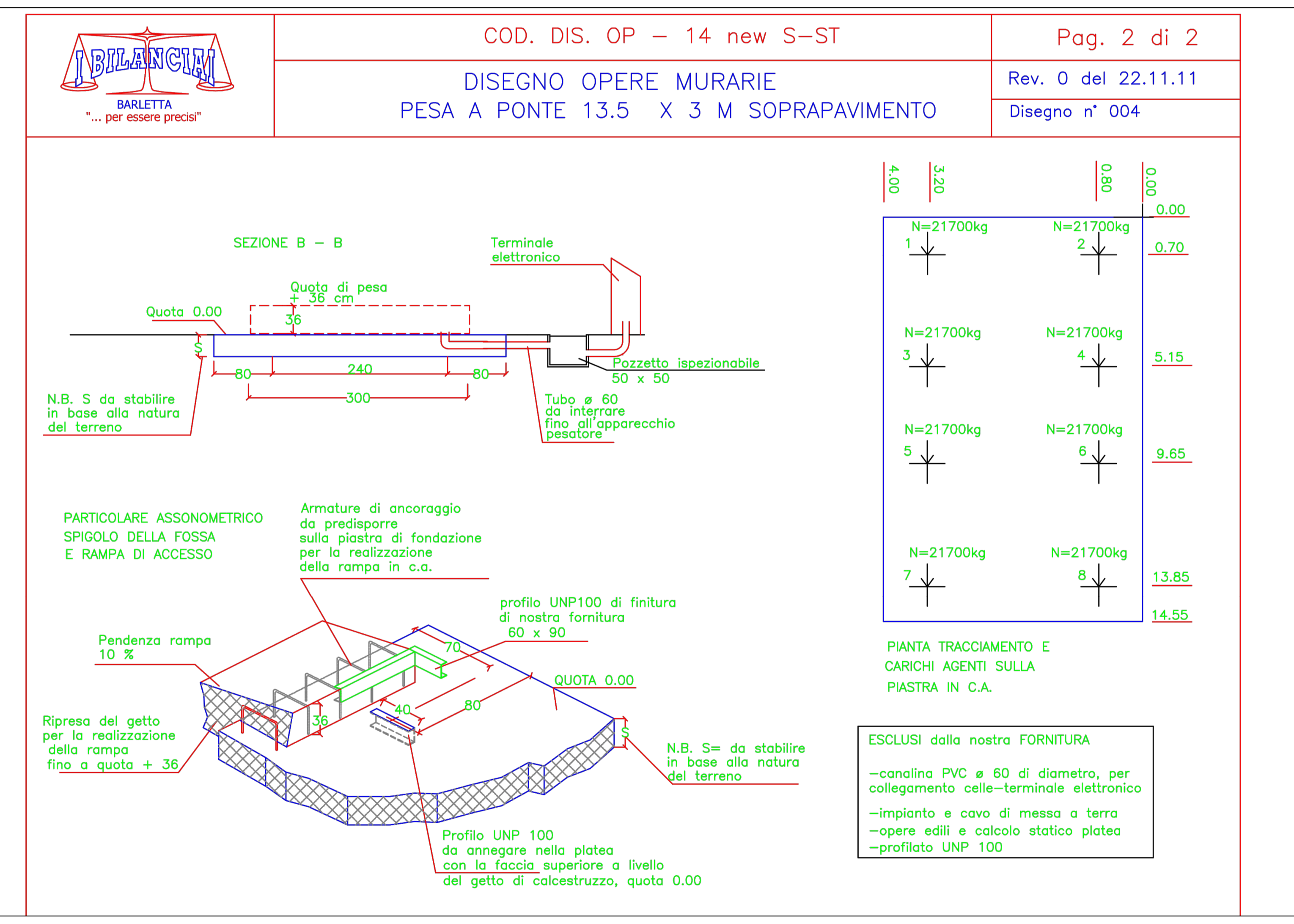
Pesa 1:50
