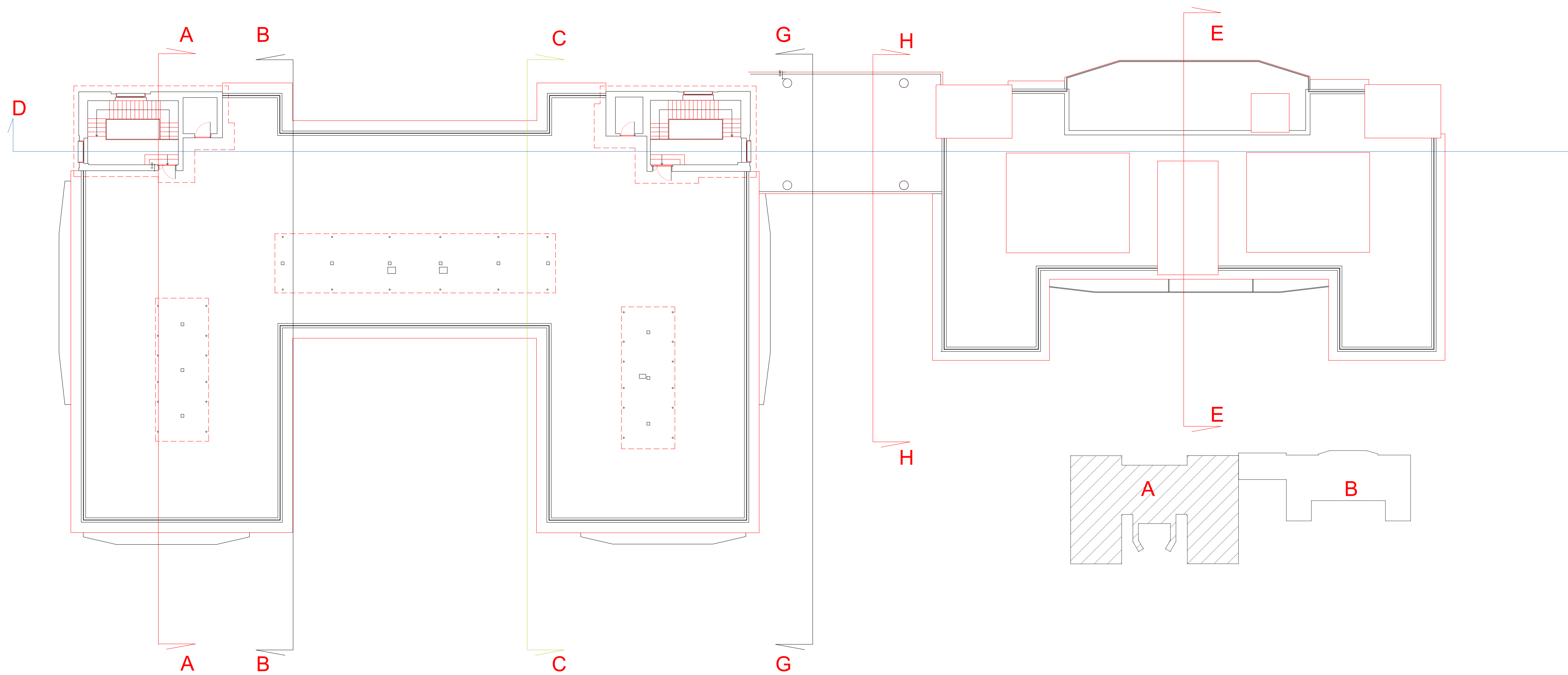
PIANTA PIANO COPERTURA
