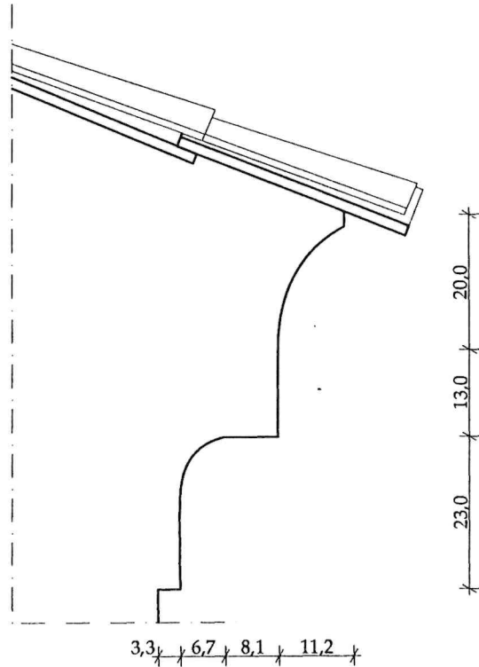
SEZIONE
