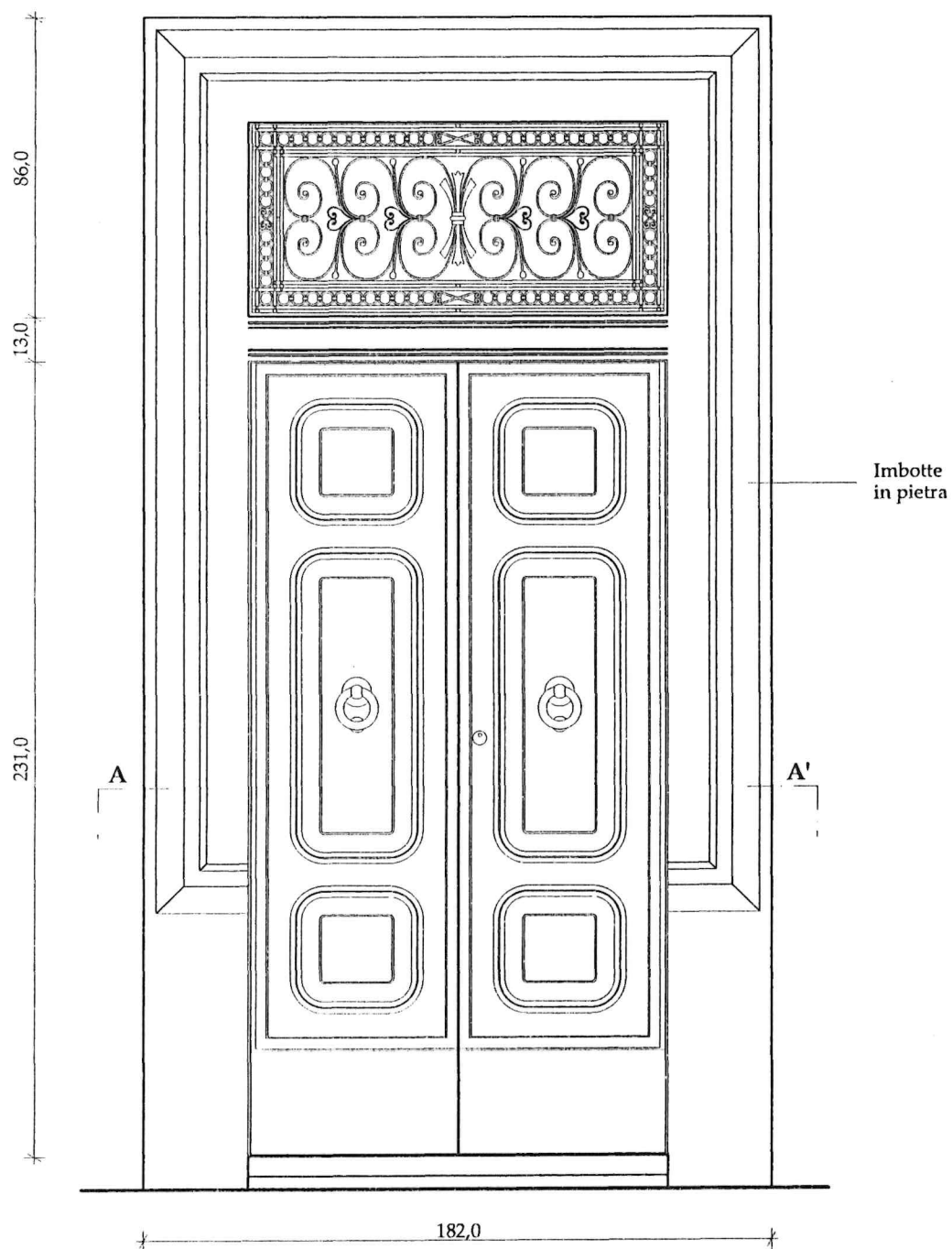
PROSPETTO ESTERNO
