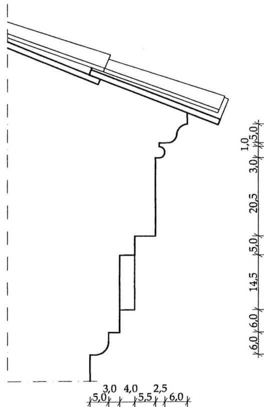
SEZIONE
