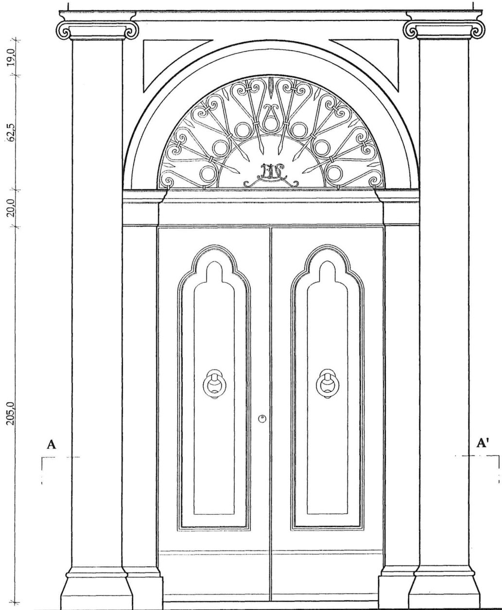
PROSPETTO ESTERNO
