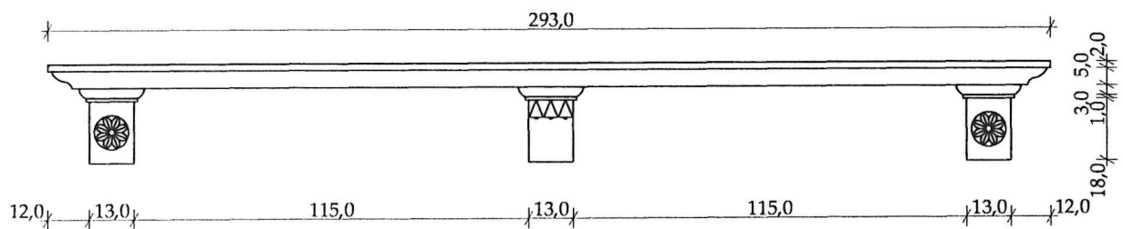
PROSPETTO FRONTALE
