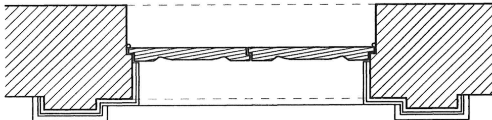
SEZIONE A-A'
