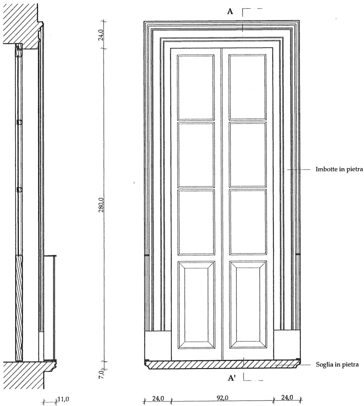
PROSPETTO ESTERNO
