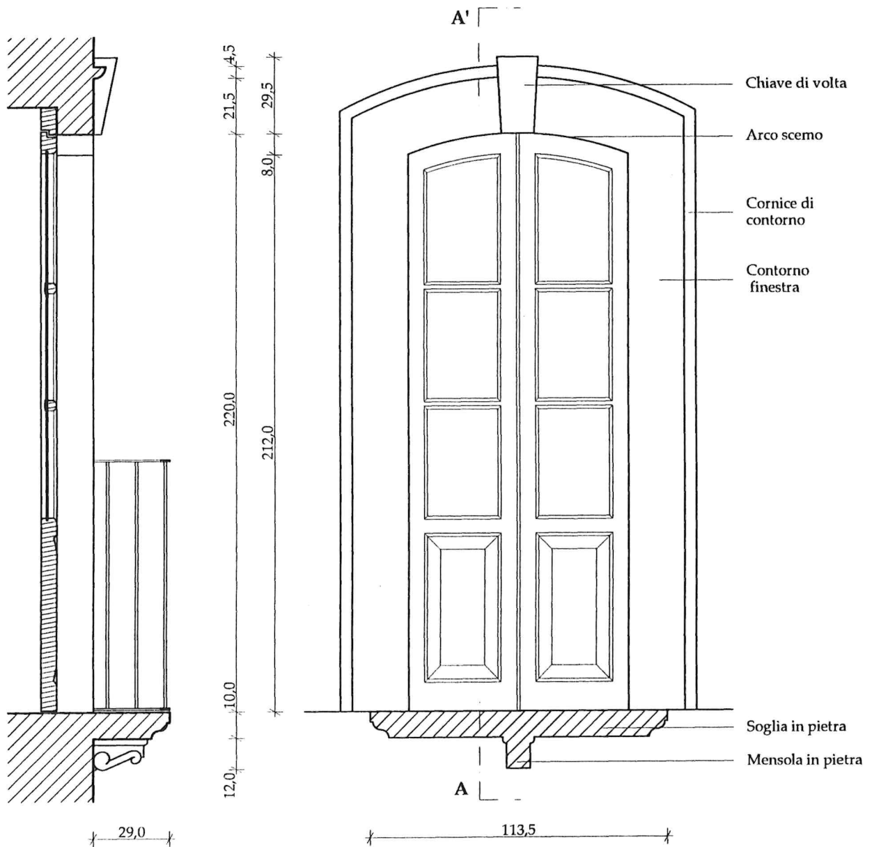
PROSPETTO ESTERNO
