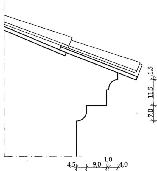
SEZIONE
