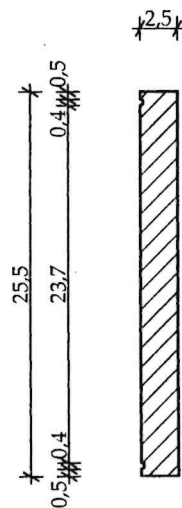
SEZIONE A-A' scala 1 : 5
