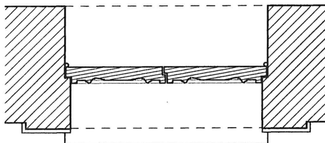
SEZIONE A-A'
