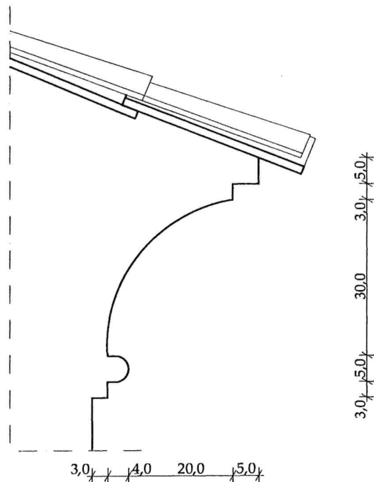
SEZIONE
