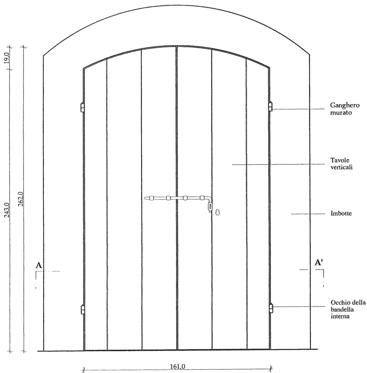
PROSPETTO ESTERNO
